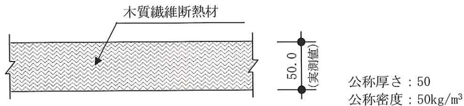
図1 試験体の断面見取り図（寸法単位：mm）
